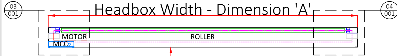
ELEVATION
